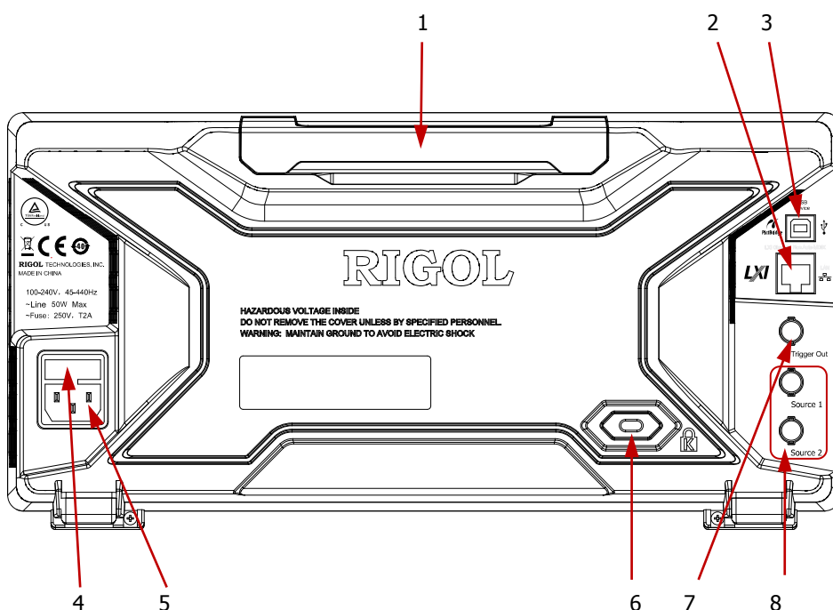
图 11 后面板总览
